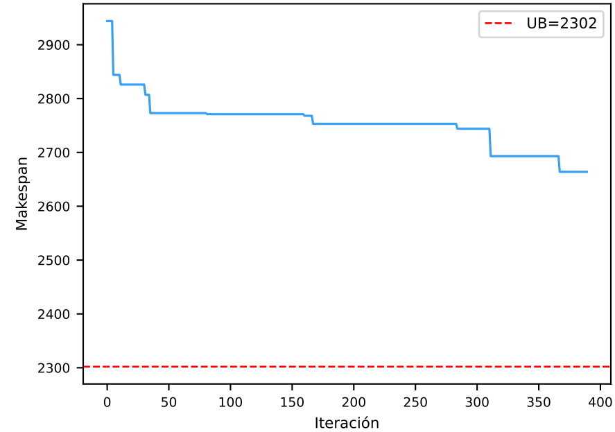
Dauzère — 13a
